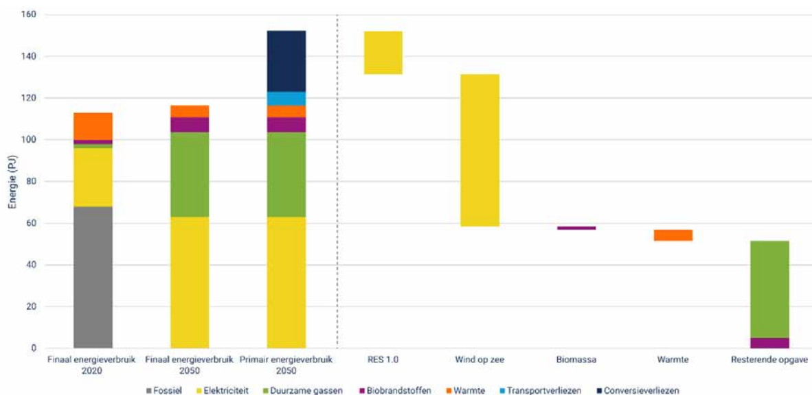
Figuur 14- Weergave van het voorziene energieverbruik (links van de stippellijn), het energieaanbod (rechts van de stippellijn) en de resterende opgave om in 2050 in de Groningse energievraag te kunnen voorzien. Hierin staan het gemiddelde finale en primaire energieverbruik 37 in 2050 op basis van de CE Delft scenario's uit de onderliggende studie. Energie is weergegeven in PJ per jaar.
