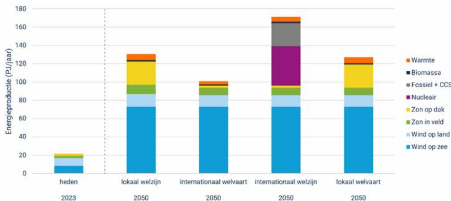
Figuren 12 en 13: Energievraag en energieaanbod in PJ per jaar in de huidige situatie en de vier scenario's voor 2050 volgens uit de CE Delft scenariostudie. Bij energievraag wordt het finaal energieverbruik 35 weergegeven. Referentie voor de huidige situatie van de energievraag is de Systeemstudie energie-infrastructuur Groningen & Drenthe door CE Delft. 36 Bij energieaanbod wordt alleen de CO 2 -vrije energieproductie weergegeven, fossiele energieproductie is dus niet meegenomen.
