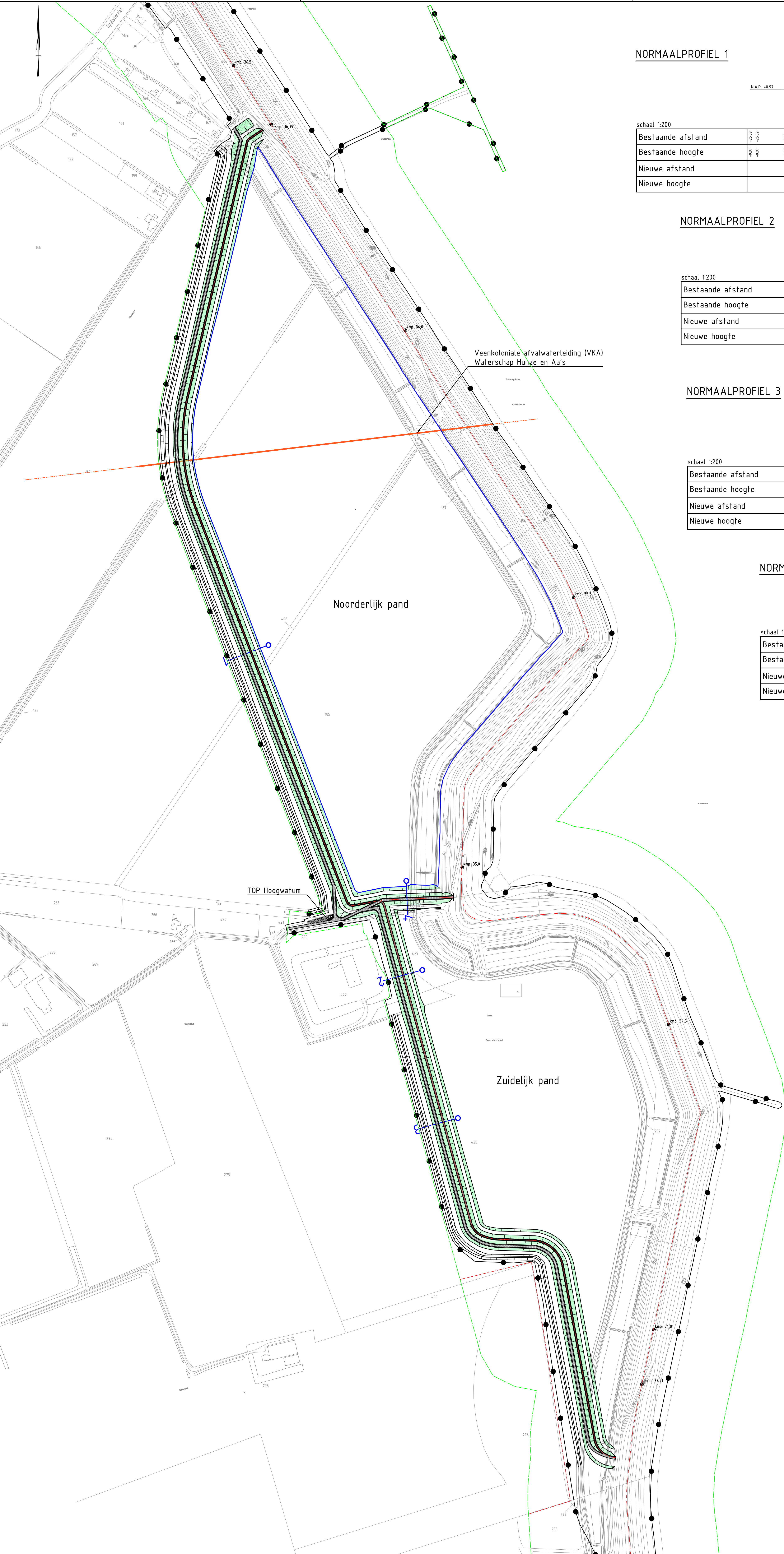
Situatie schaal 1:2.500
